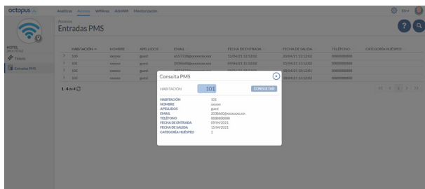
Imagen 5. PMS inquiries
